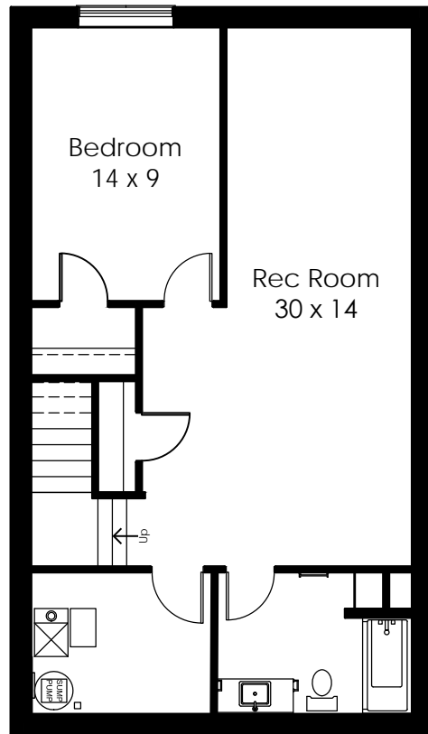
Optional Basement Plan 682 sqft
